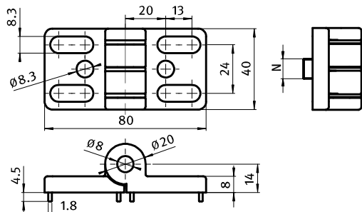
Zinkdruckguss-Scharnier Zinc Die-cast Hinge
