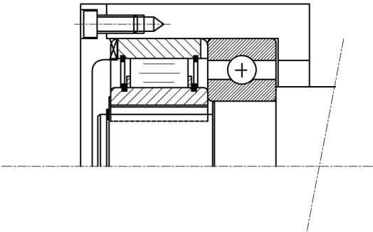
Esempio di montaggio Mounting example Exemple de montage
