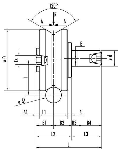
ROTELLE SCANALATE - GROOVED WHEELS - ROULETTES RAINURÉES FIG. 1
